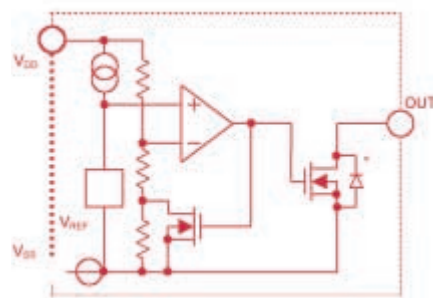
S-808xxC (utan tillslagsfördröjning)
