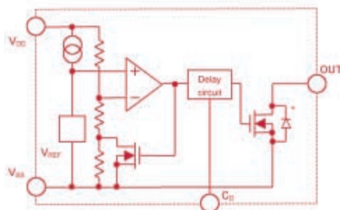
S-809xxC (med tillslagsfördröjning)
